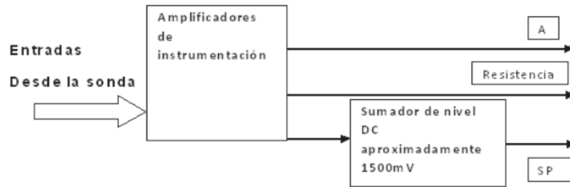
Figura7. Diagrama de bloques general del acondicionador de señal
