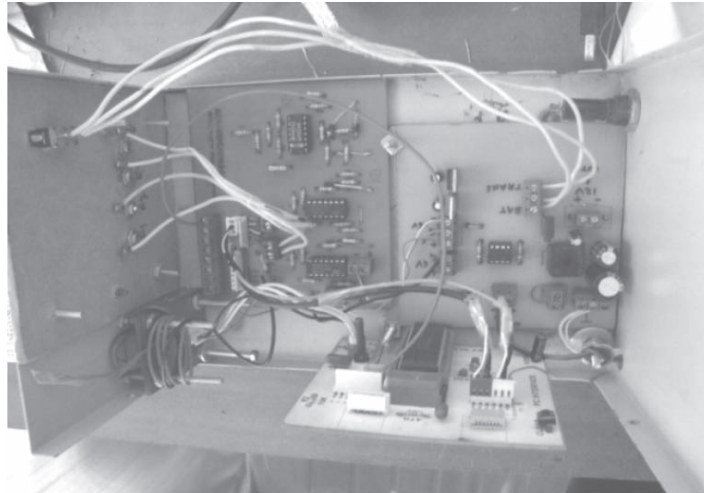
Figura 10. Vista interna del hardware del proyecto
