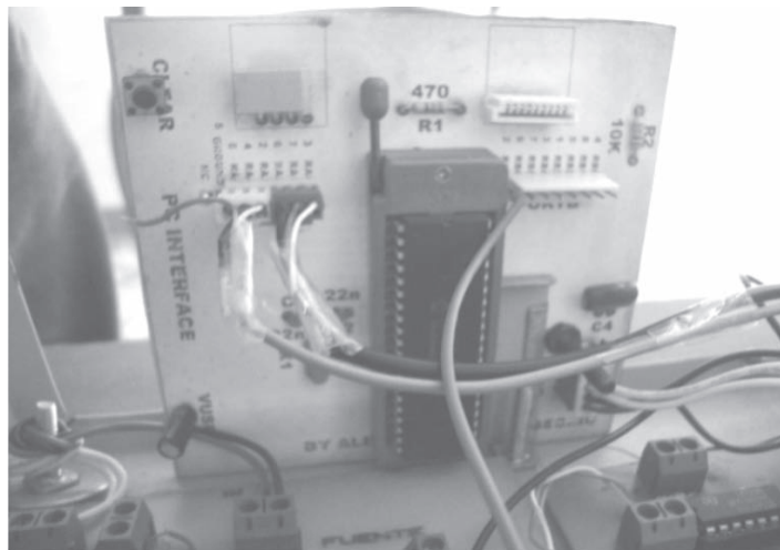
Figura 11. Etapa de adquisición de datos
