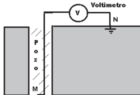
Figura 1. Esquema para medir SP
