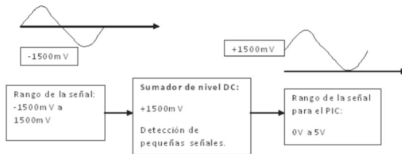
Figura 6. Suma de nivel DC para medición de SP
