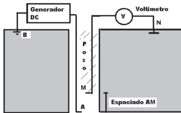
Figura 2. Esquema para medir resistividad
