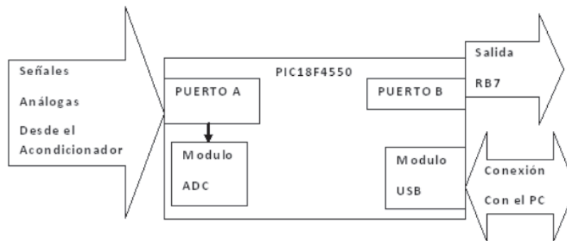
Figura 8. Diagrama de bloques de la tarjeta de adquisición de datos
