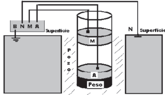
Figura 5. Vista interna de la sonda y conexión al dispositivo de medición
